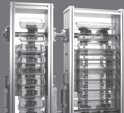
アルミ製ゴルフボール縦型コンベアー（T3/T6）
